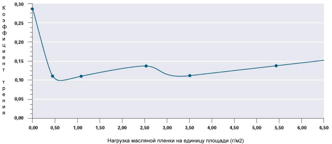
Коэффициент трения как отличительная особенность масляной пленки жидкостей на основе растворителей
